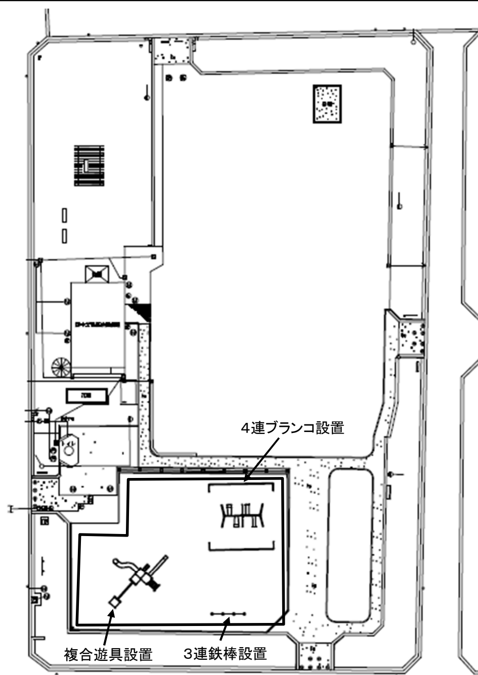
< 計画平面図 >
