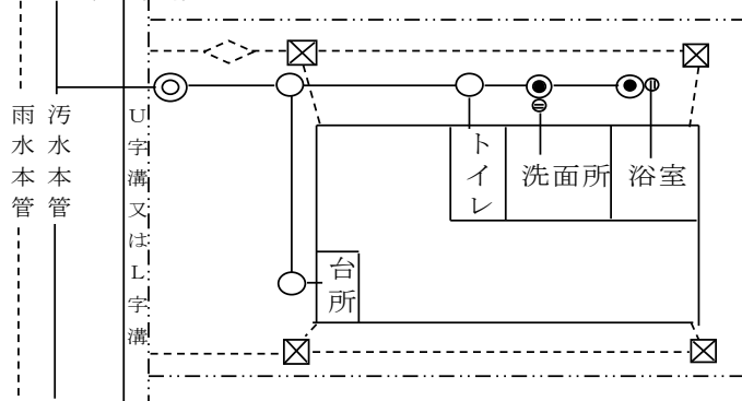
(屋外排水設備の例)
