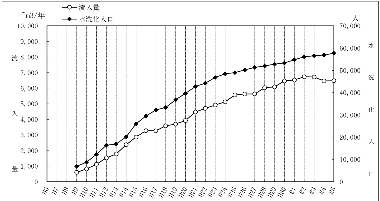
流入量と水洗化人口の推移
