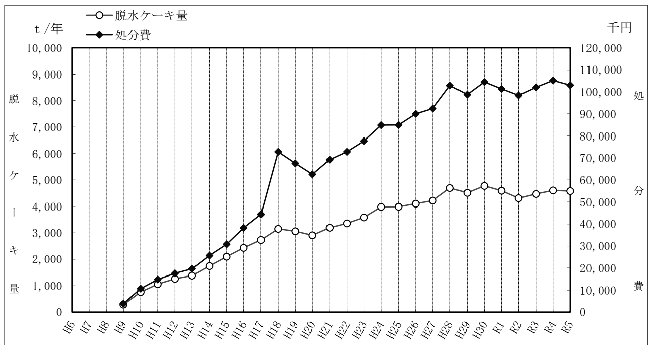
脱水ケーキ量と処分費の推移
